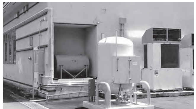
ふれあい館バルクガスタンク
